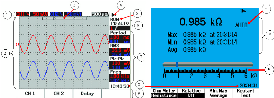
Figure 1 Affichage d'oscilloscope
